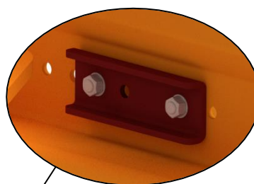
Contraplaatje van de aanbouwdelen (4 stuks benodigd)
