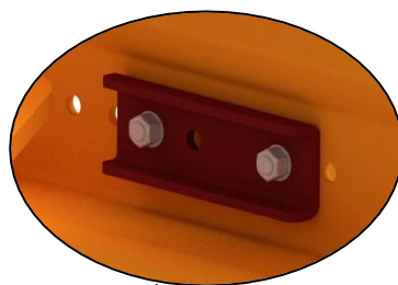
contraplaat voor de aanbouwdelen (vier stuks benodigd)
