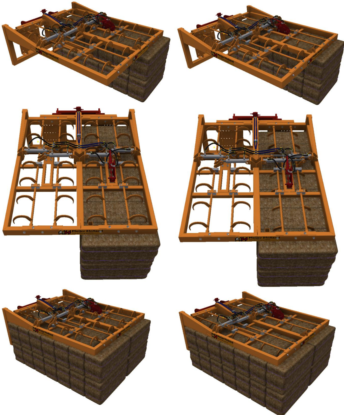
beweging klemhaken
